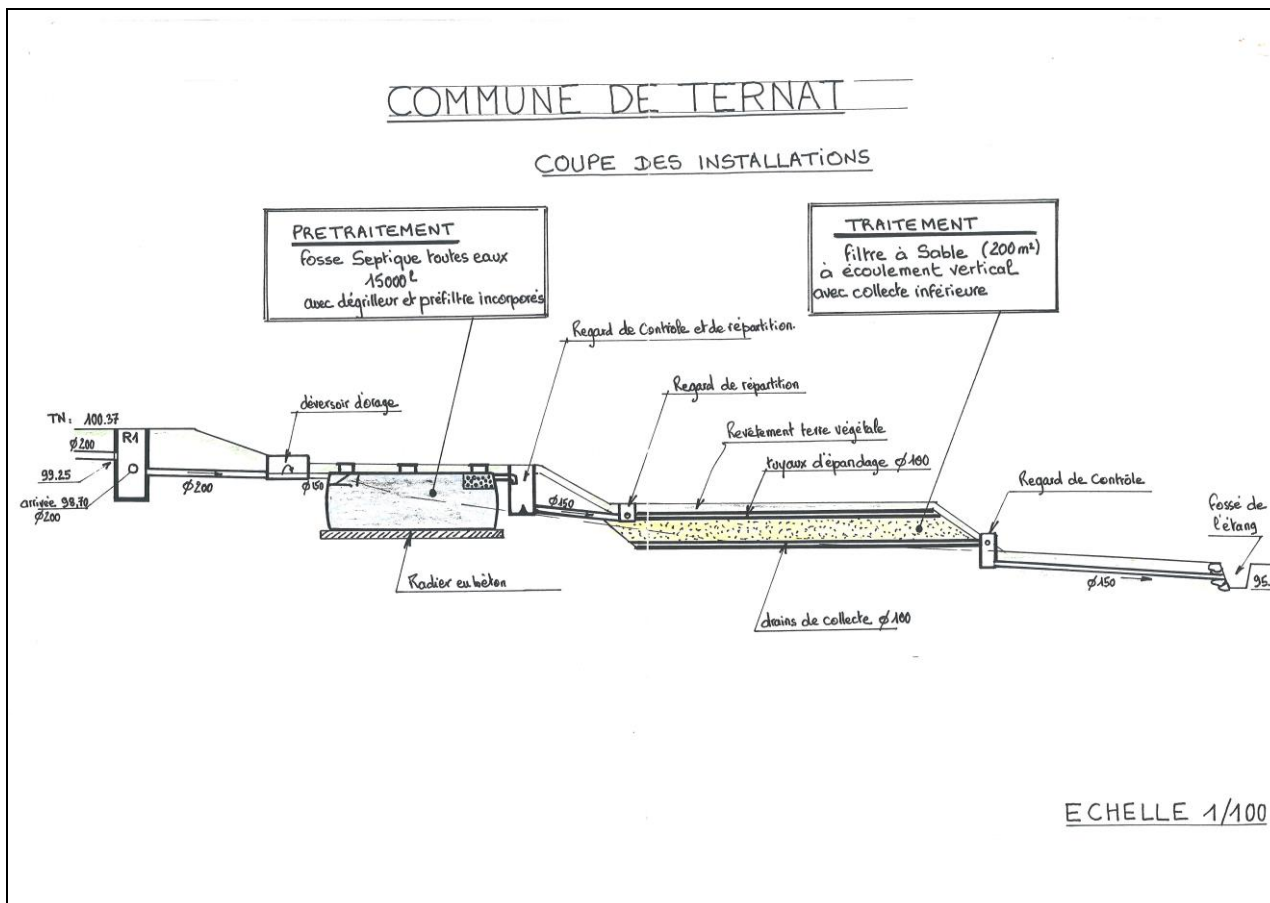
Station d'épuration de Ternat : filtre à sable drainé
