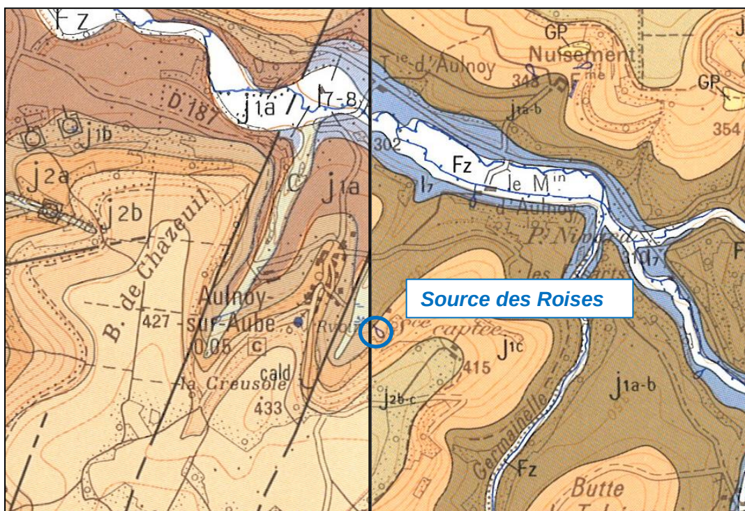
Extrair des carres géologiques 1/50000 du BRGM « RECEY-SUR-OURCE et LANGRES »
